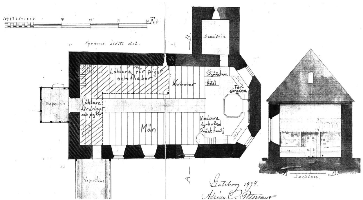
Bild nr. 3 Ritning över Ornunga gamla kyrka kopierad från original hämtad vid Göteborgs landsarkiv. Bänklaceringen inritad efter Marianne Lindhs beskrivning.
